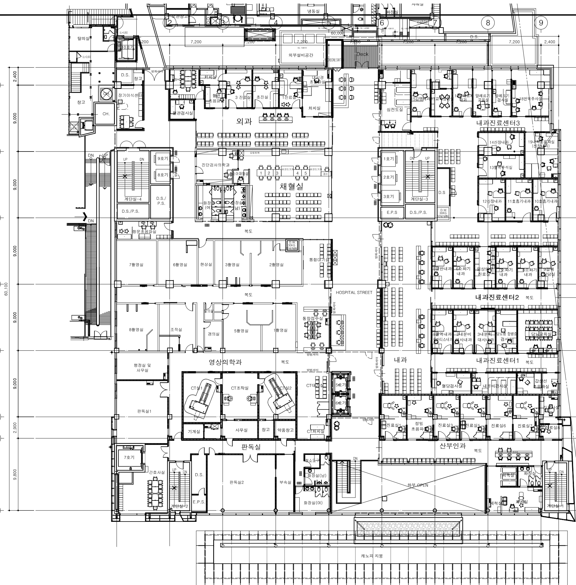
1 2층 평면도 축척 : A1: 1/150 A3: 1/300 면적=3,652.73m2
